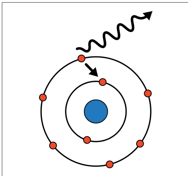
Abb. 3: Bewegung eines Elektrons unter Freisetzung von Energie/Photon
