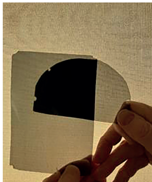
Abb. 8 u. 9: Keine Lichtabsorption bei parallelen Polfiltern. Lichtabsorption durch zwei Polarisationsfilter, die im 90° Winkel zueinanderstehen.
