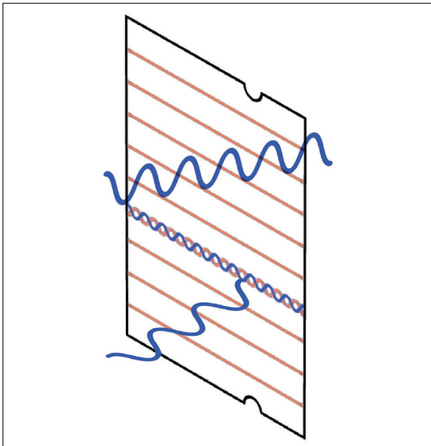
Abb. 7: Polarisationsfilter. Die parallelen Polymerlamellen sind braun horizontal eingezeichnet. Die horizontal eintreffende elektromagnetische Welle (die im Bild untere) wird gelöscht, da sie mit den Polymeren interagiert. Die vertikal eintreffende (im Bild die obere) interagiert nicht und passiert den Polarisationsfilter.
