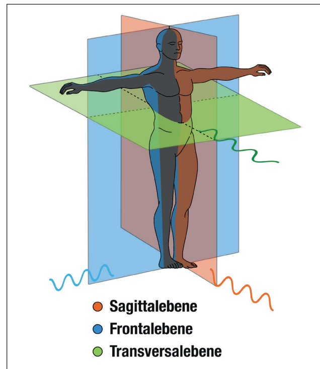
Abb. 2: Die Richtung der elektromagnetischen Wellen als Vektor der elektromagnetischen Felder
