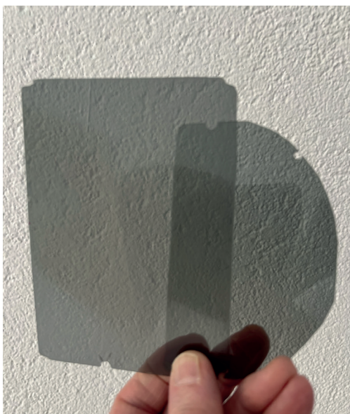
Abb. 8 u. 9: Keine Lichtabsorption bei parallelen Polfiltern. Lichtabsorption durch zwei Polarisationsfilter, die im 90° Winkel zueinanderstehen.
