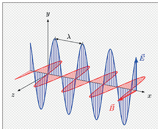
Abb. 5: Linear polarisierte elektromagnetische Welle im Vakuum ( https://de.wikipedia.org/wiki/Elektromagnetische_Welle )
