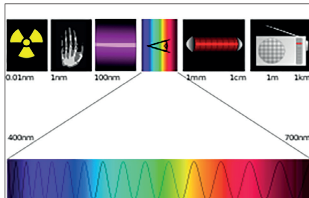
Abb. 6: Elektromagnetisches Spektrum. Die Energie der elektromagnetischen Wellen ist proportional zu ihrer Frequenz.
